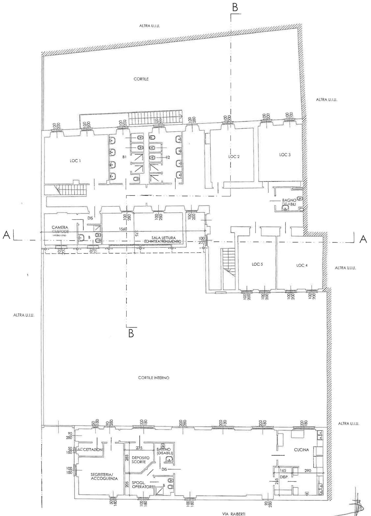
PIANTA PIANO TERRA - PROGETTO
