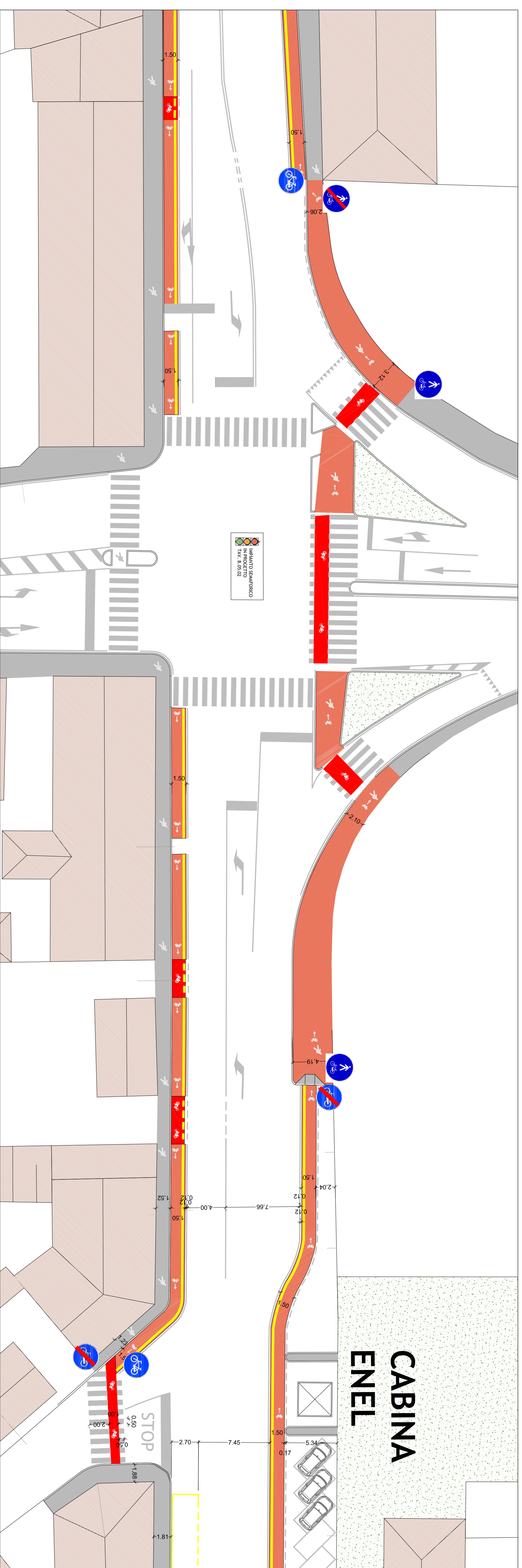
Planimetria di PROGETTO - RIQUADRO 03 Sc. 1:200
