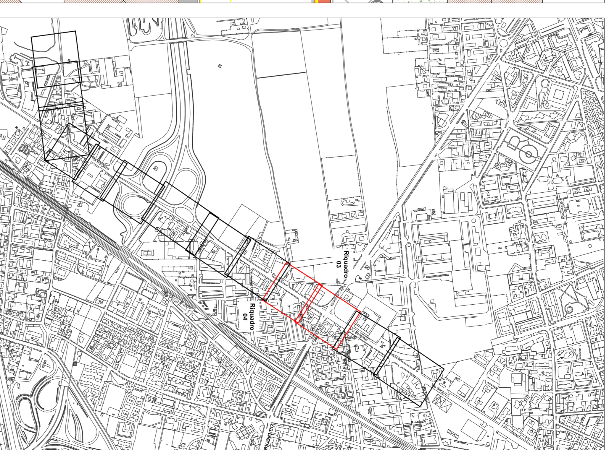
Estretto di Fotogrammetrico Sc. analitica
