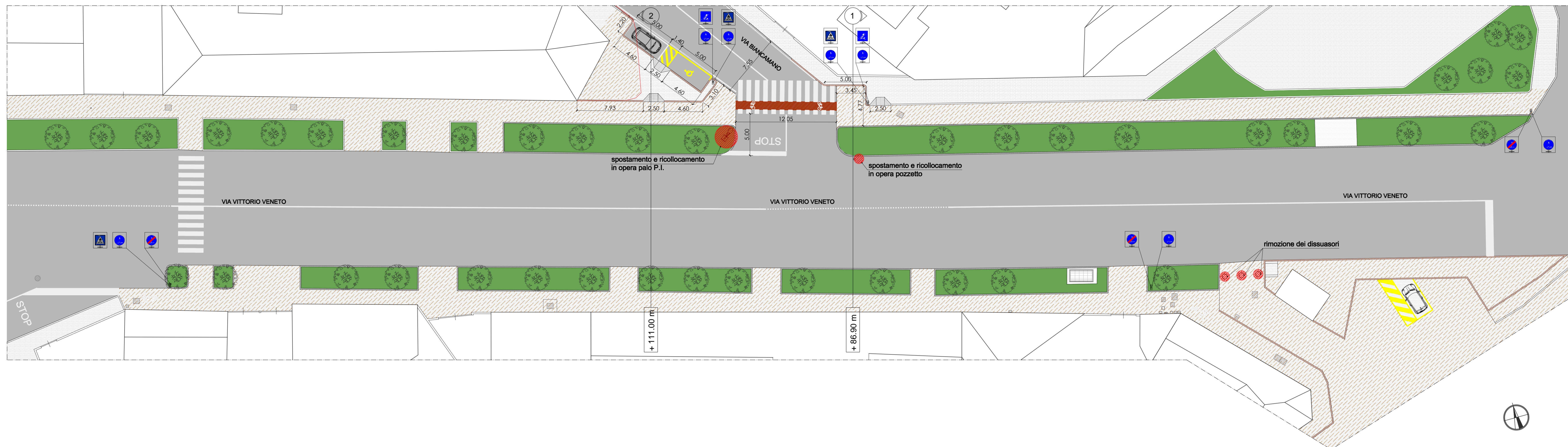
Planimetria di progetto - scala 1:200
