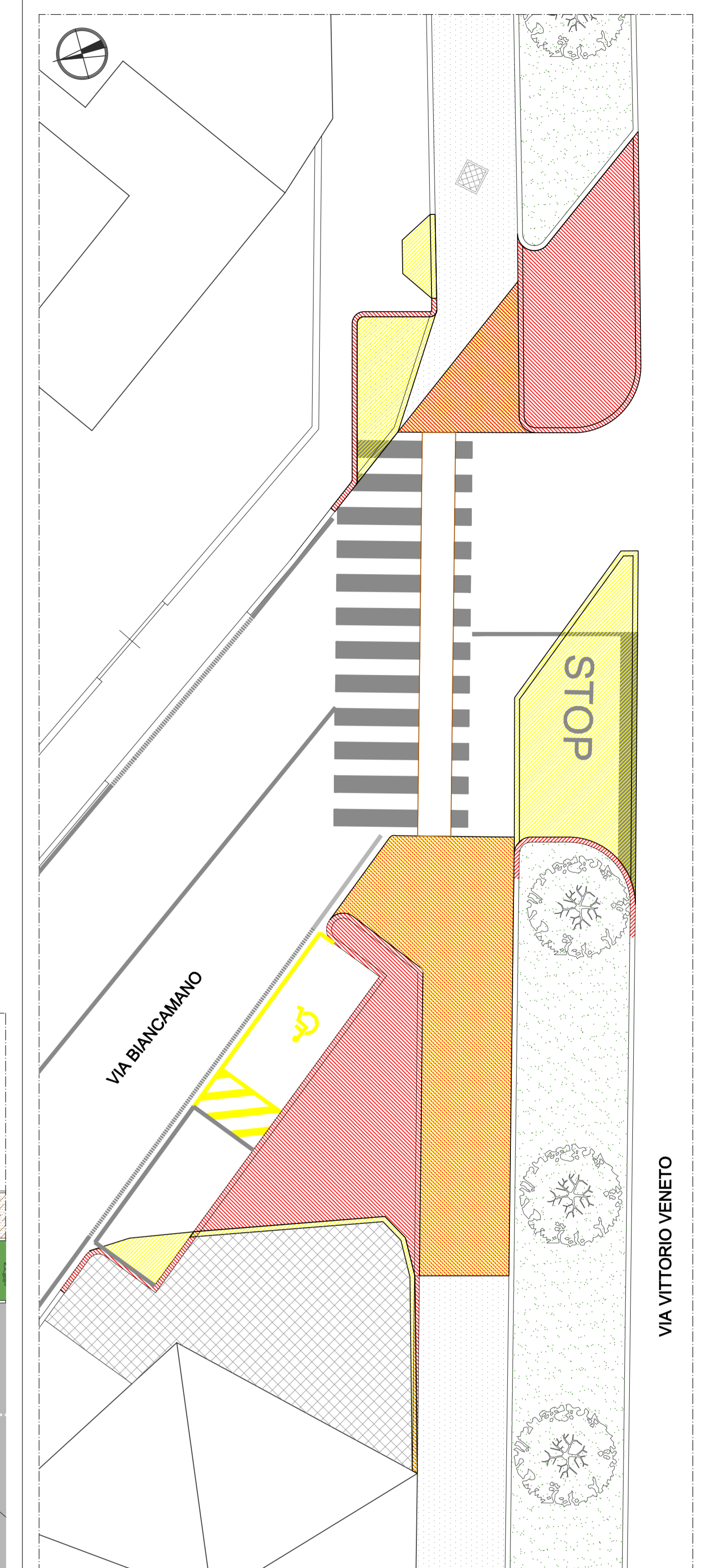
Planimetria di progetto con evidenziazione delle principali lavorazioni - Incrocio con via Biancamano - scala 1:100
