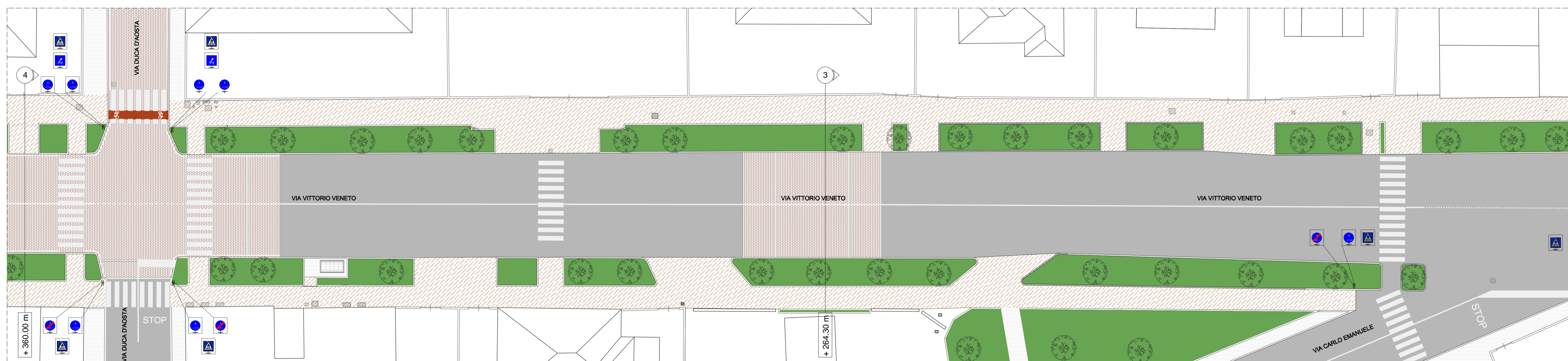
Planimetria di progetto - scala 1:200
