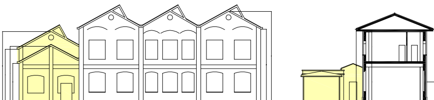
SEZIONE K-K'
