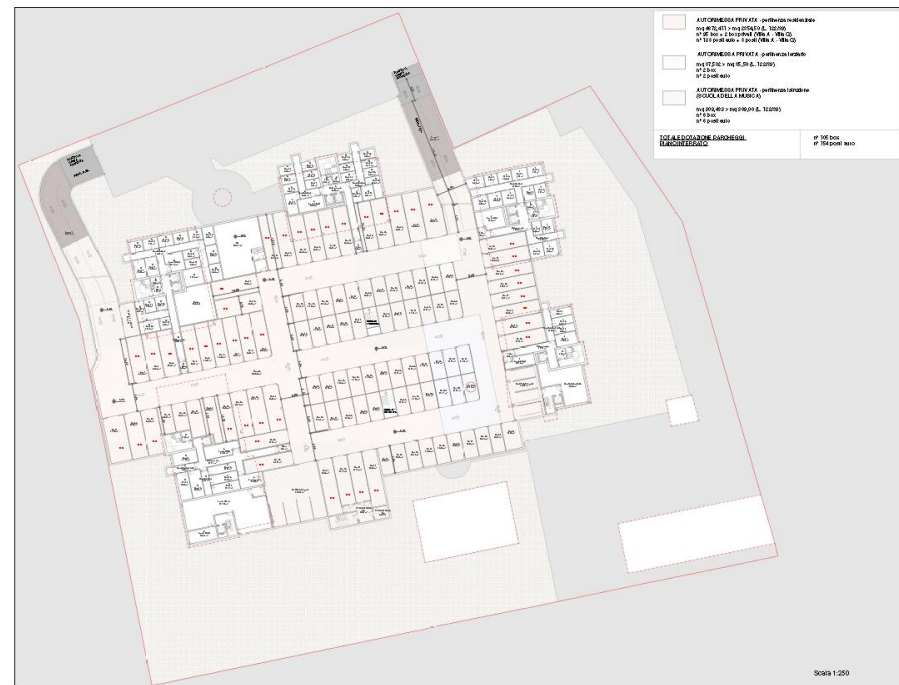
Figura 65 – Planimetria di progetto P.I.I. ex Feltrificio Scotti – Piano interrato
