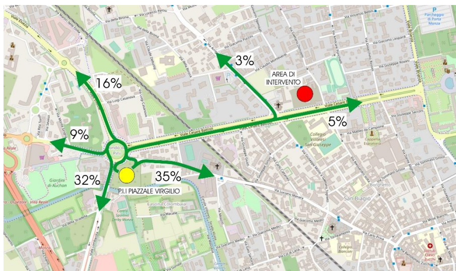
Figura 55 – Itinerari di distribuzione traffico indotto in uscita – P.I.I. piazzale Virgilio
