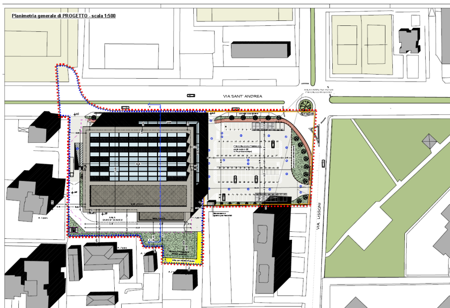
Figura 41 – Planimetria intervento P.A. ex Cinema Maestoso
