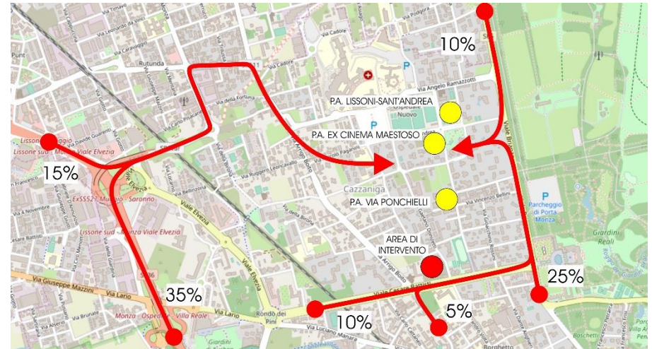
Figura 52 – Itinerari di distribuzione traffico indotto in ingresso – P.A. Lissoni-Sant'Andrea, ex Cinema Maestoso e via Ponchielli
