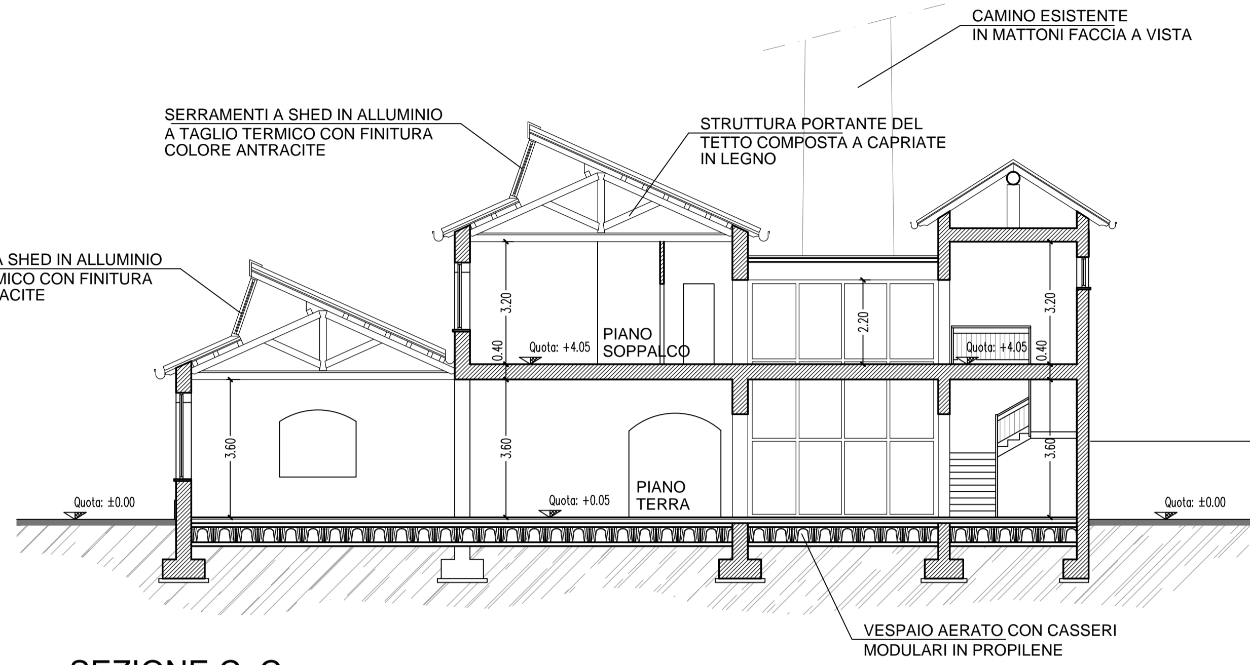
SEZIONE C+C
