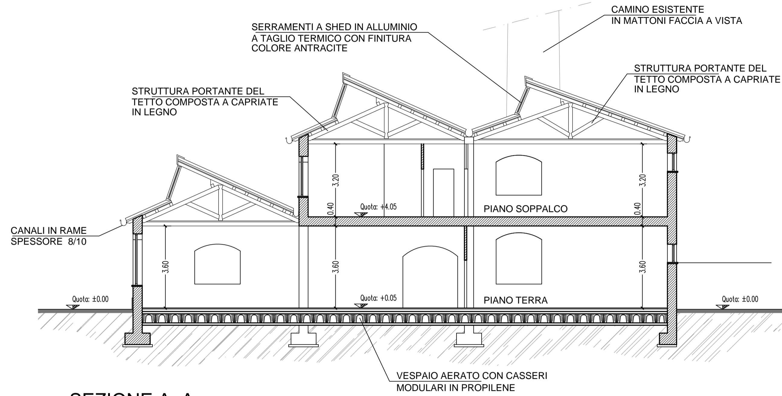
SEZIONE A+A
