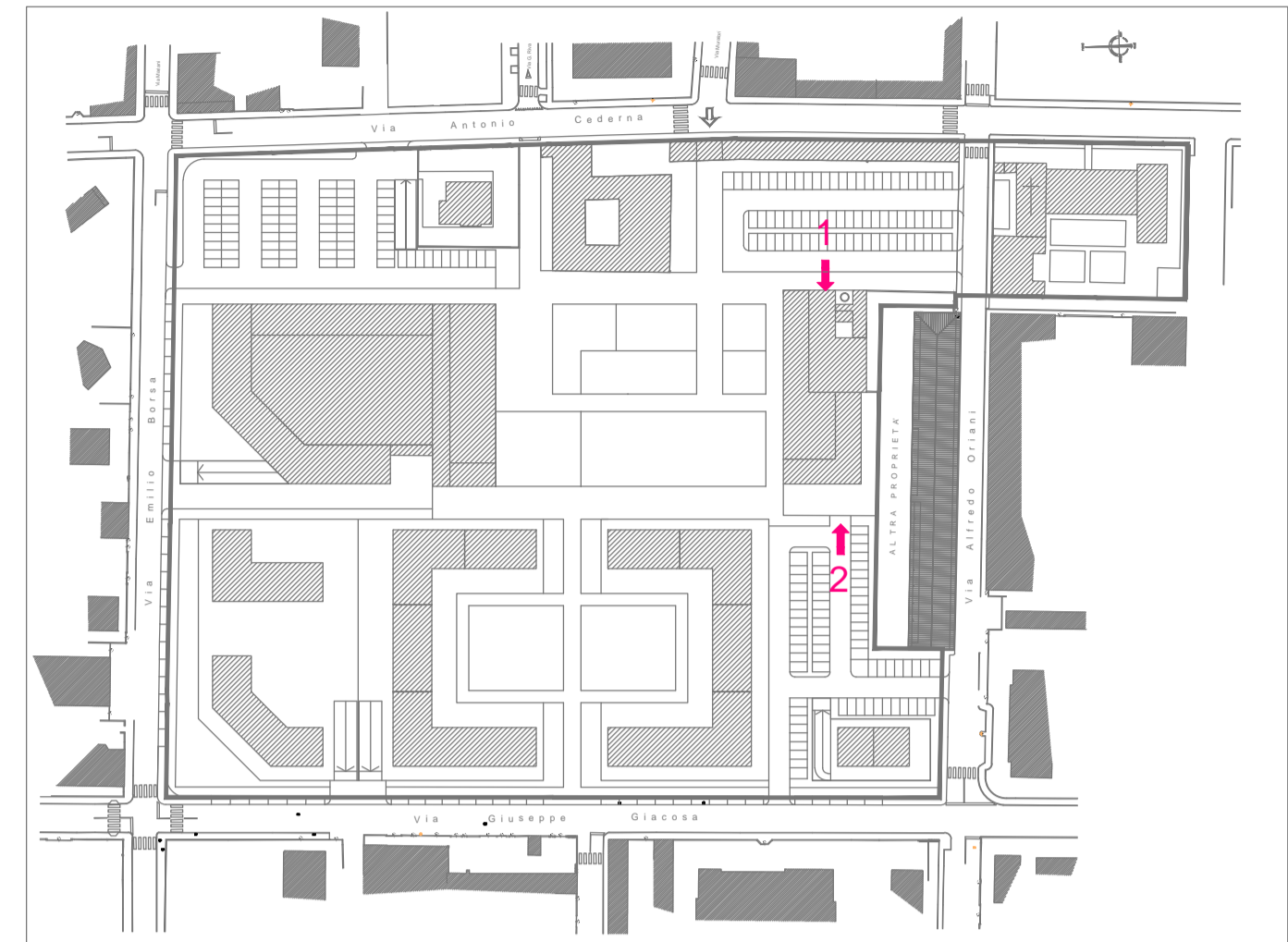
SCHEMA DEGLI ACCESSI ALL'EDIFICIO PUBBLICO 1 - ACCESSO PEDONALE 2 - ACCESSO CARRAIO E PEDONALE
