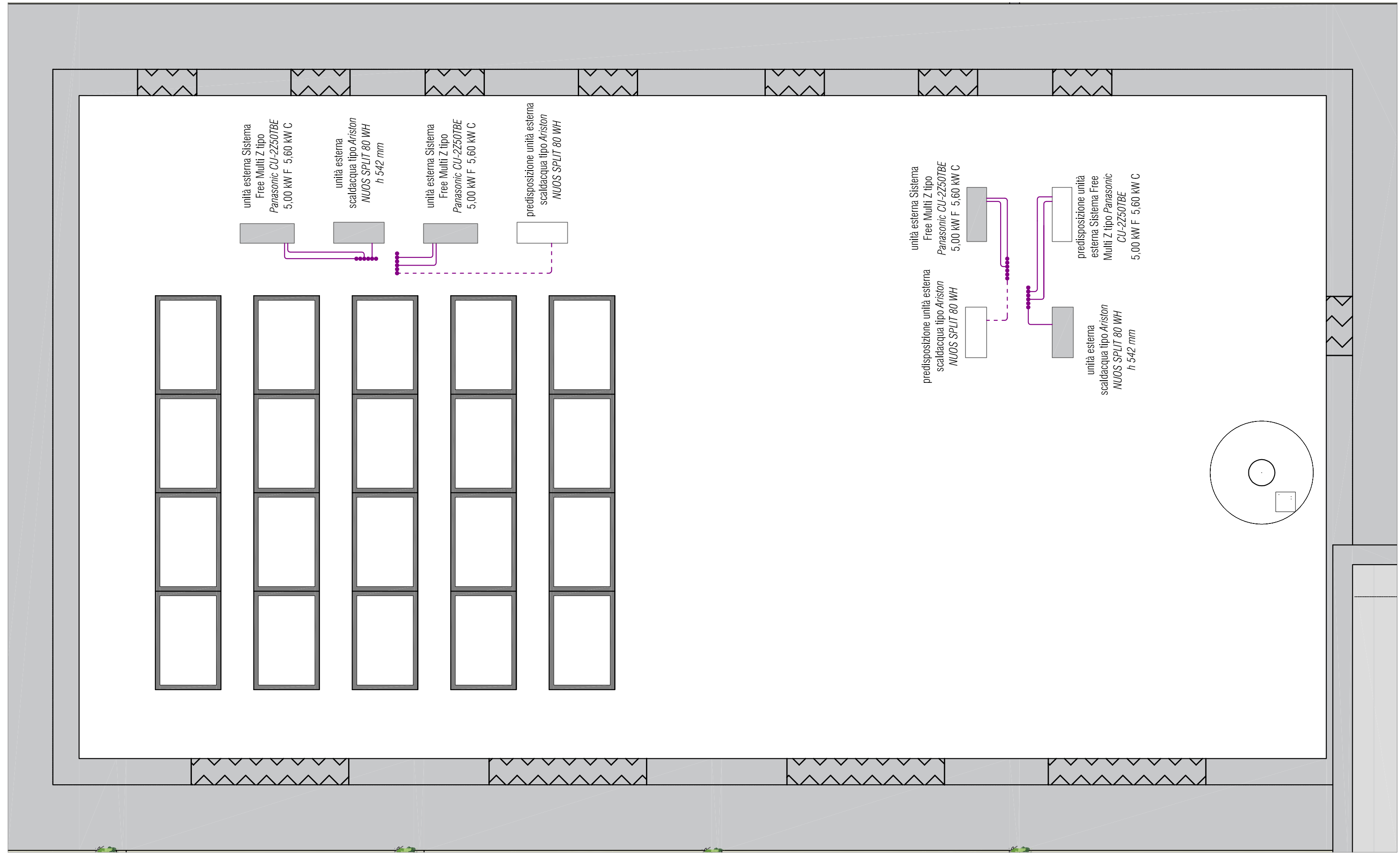
COPERTURA - scala 1:50
